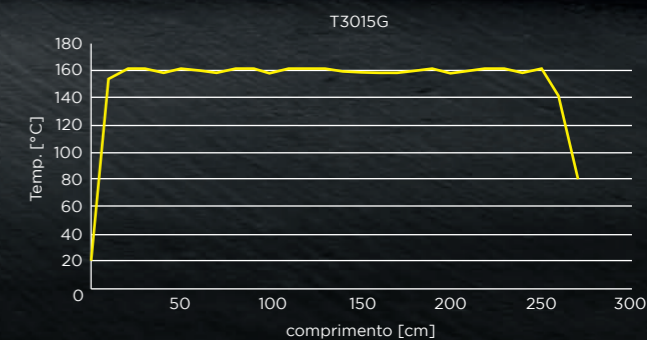
DISTRIBUIÇÃO DO CALOR DENTRO DE UMA ROQ SAHARA
